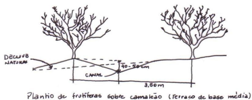
Figura 34 - Corte de um terraço, mostrando sua localização, bem como a do canal
